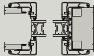
Telaio in alluminio Classic "SeEven". Anta singola scorrevole a scomparsa, con profilo in alluminio e doppio vetro. Mod. ACIDATO
