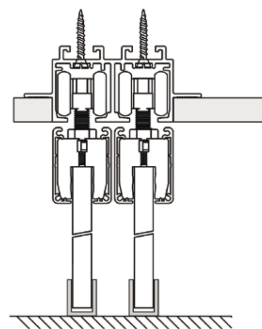
Sistema Scorrevole Con Binario A Scomparsa "TSC200" due o quattro ante parallele con anta fissa
