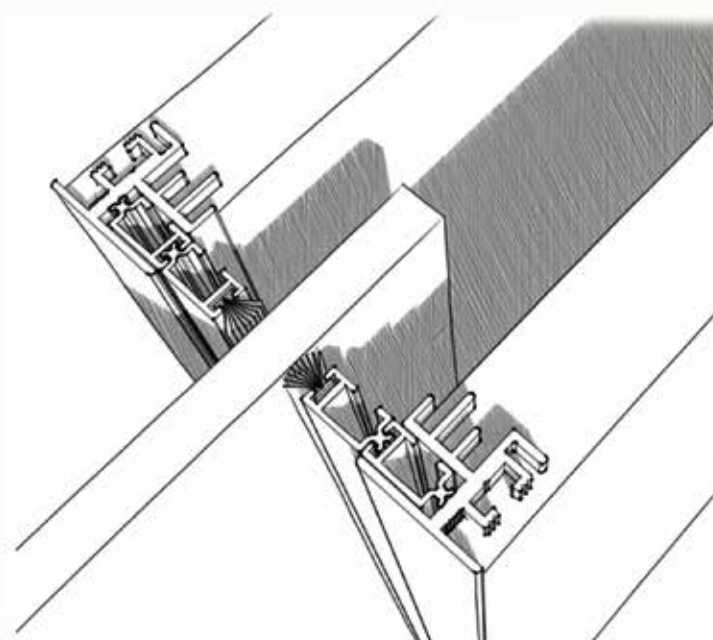
Scorrevole a scomparsa "MODULAR RASO" Telaio senza mostre da rasare adattabile a controtelai standard Anta singola Mod. Trasparente_Collezione TRASPARENTI
