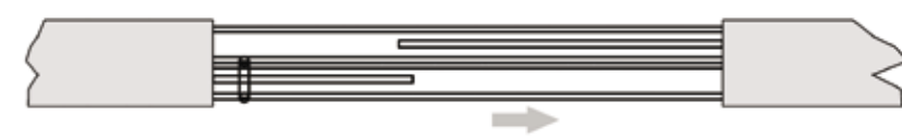
Sistema scorrevole con binario a scomparsa "SVF150TM" Anta scorrevole e anta fissa
